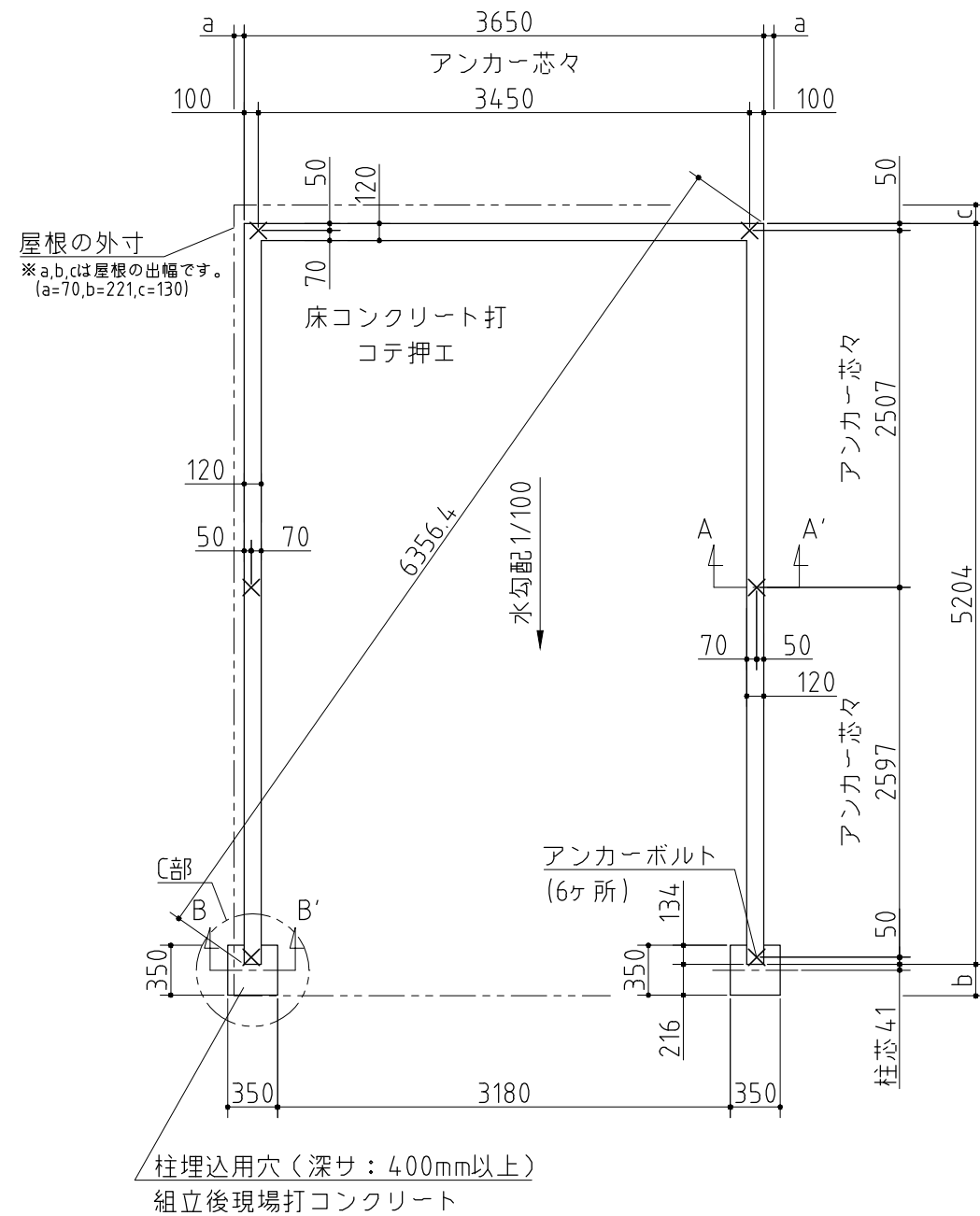
基礎詳細図 S=1/20
